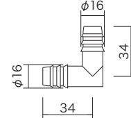
FDエルボコネクタ
