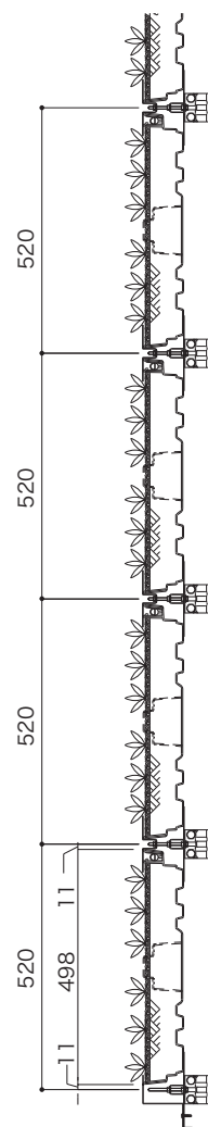
A断面 (山部)
