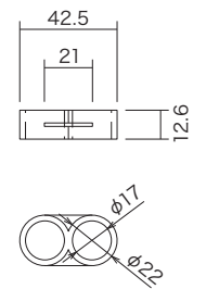
FDラインエンド
