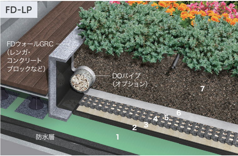
仕様構成部材(1、7は価格別途)
