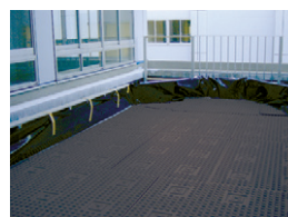
FDドレインLN設置
