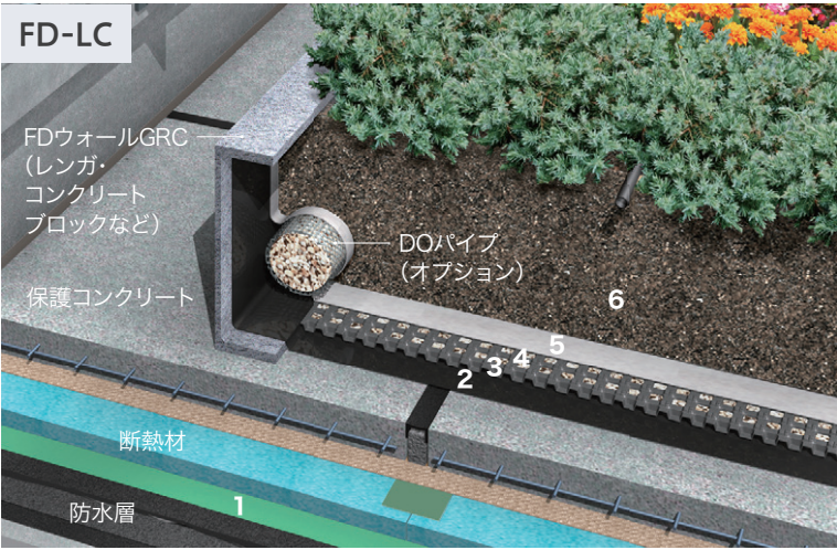
植栽見切材(例)
