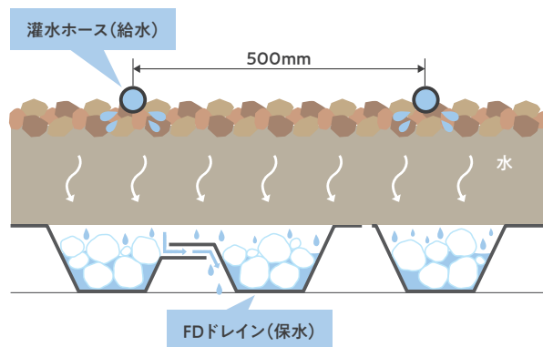
ドリッパー詳細図
