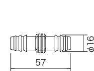
FDチューブコネクタ
